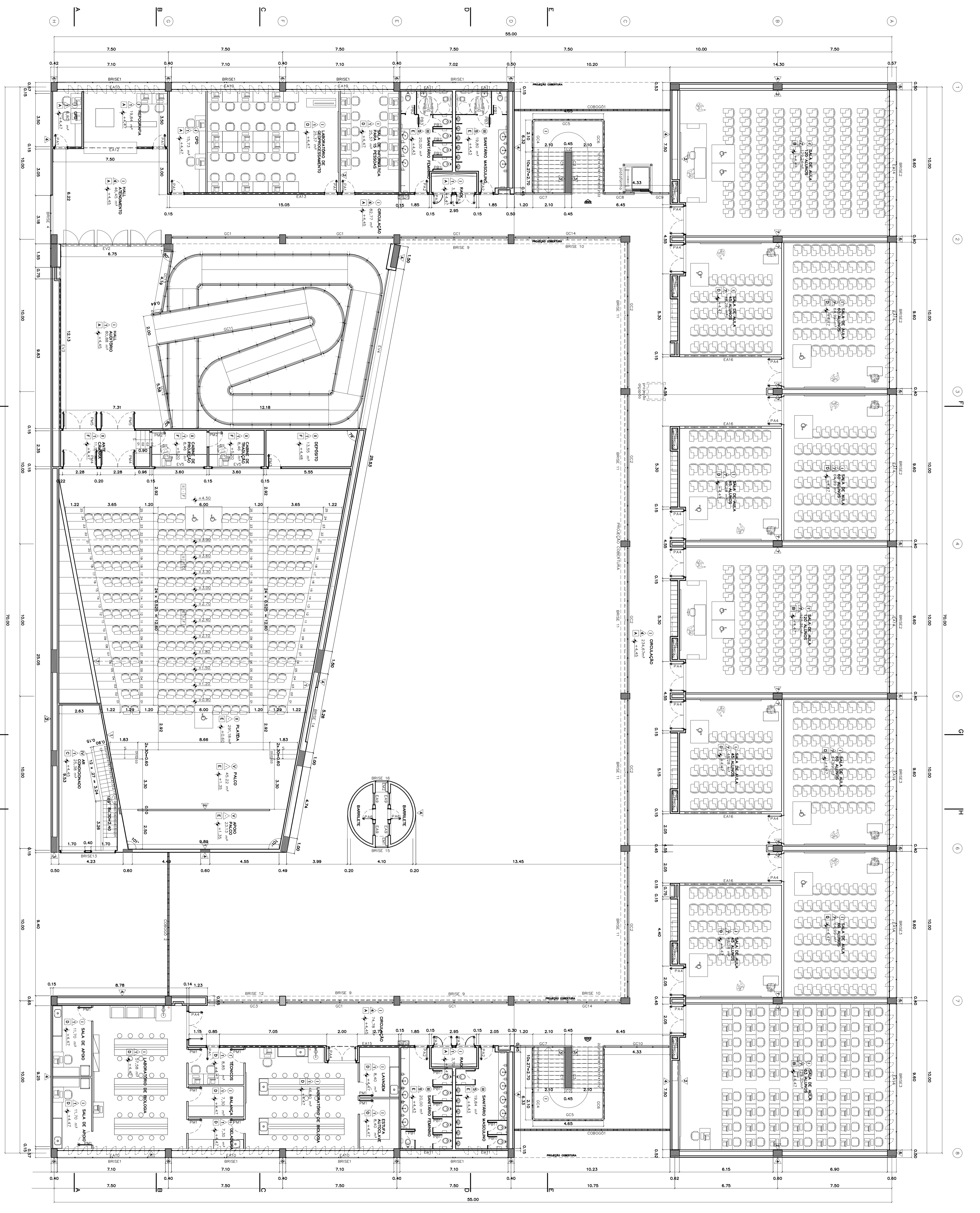
PLANTA PAVILÃO SUPERIOR Escala: 1:100 Data: 20/05/2010
