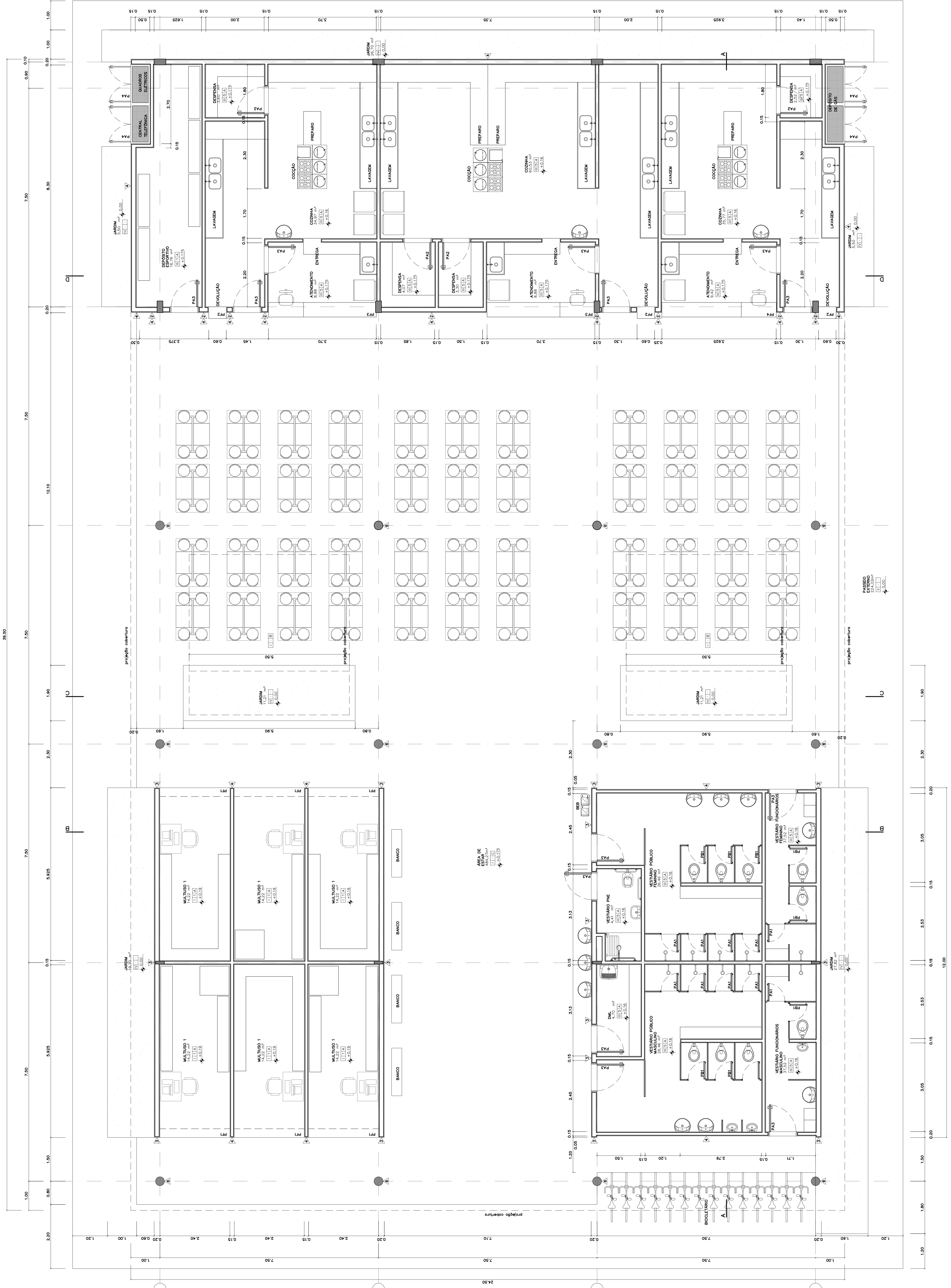
PLANTA BAIXA ESC. 1/50 MAR/2014
